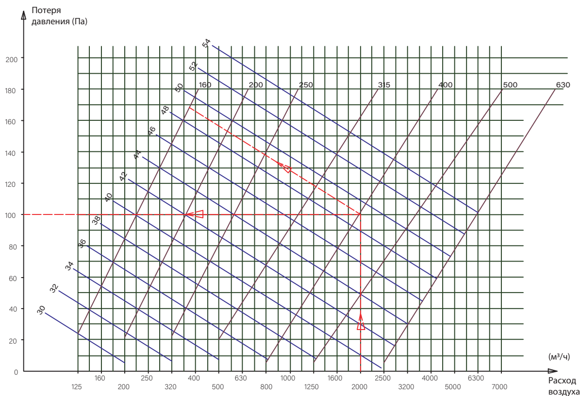
Кривая зависимости расхода воздуха, потери давления и уровня шума для серии JVA ( V_x = 0,5 м/с).
