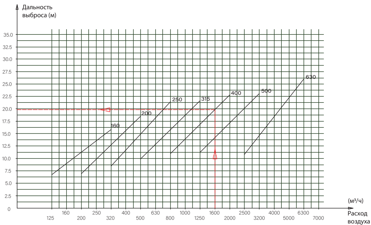
Кривая расхода воздуха и дальности выброса для серии JVA ( V_x = 0,5 м/с).
