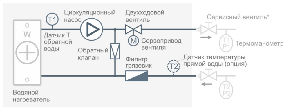
Схема смесительного узла с двухходовым вентилем
