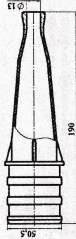
Тип 2 (конструктивный вид -01)
